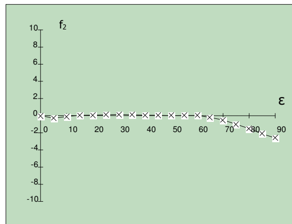
Bild 3: typische Abweichung der räumlichen Bewertung f_2 ( \epsilon )
