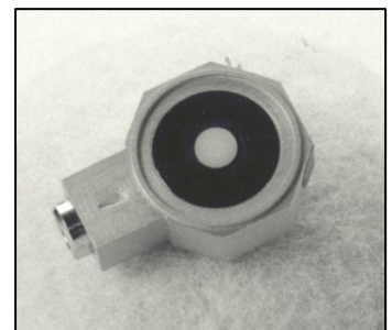
Bild 8: Mini-Photometerkopf
